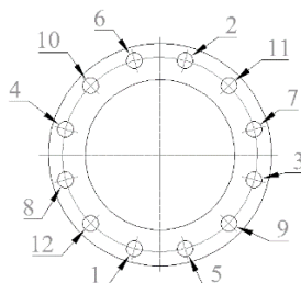
Rysunek 4. Kolejność dokręcania nakrętek.
