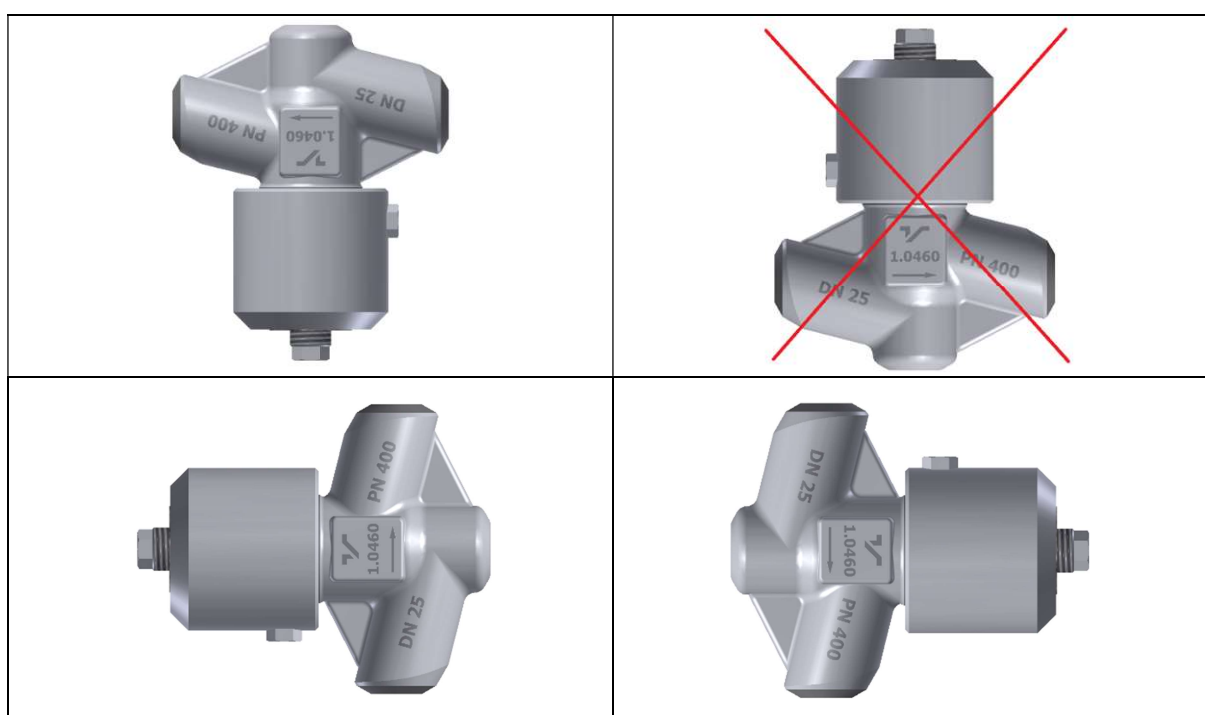
Rysunek 2. Zalecana pozycja montażu
