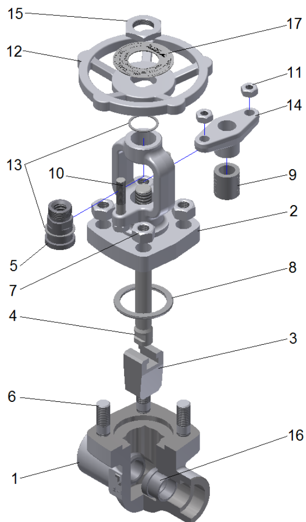
Rysunek 1. Części składowe zasuw
