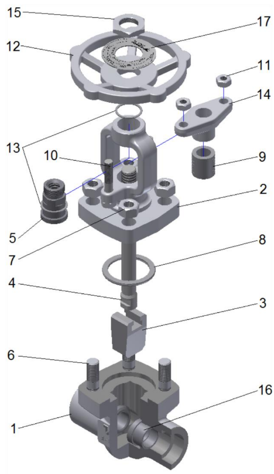
Rysunek 1. Części składowe zasuw
