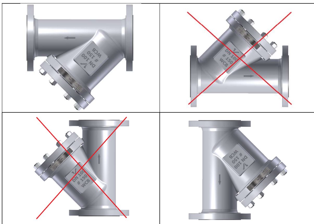
Rysunek 2. Zalecana pozycja montażu
